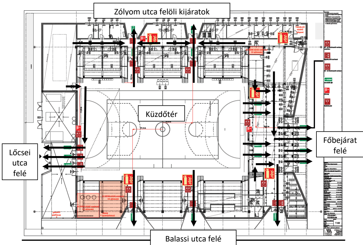
Földszint
